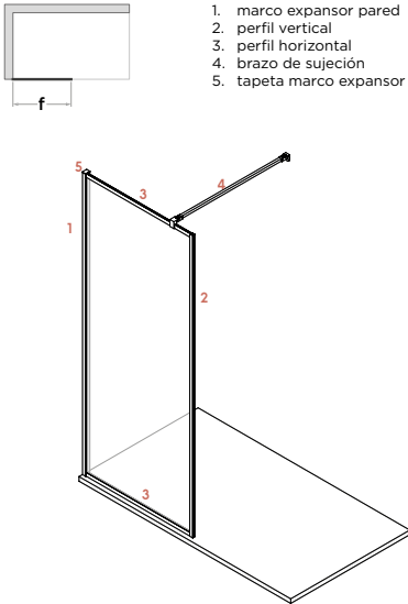
Frontal 1 hoja fija
