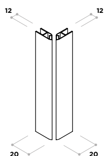
02020001 02020019 Cierre de imán angular 90°
