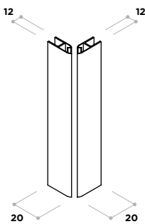
02020001 Cierre de imán angular 90°
