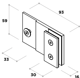
02010639 Soporte guía-fijo lateral Océanos Aluminio
