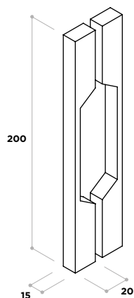
02010382 Tirador cube 20 Zamak
