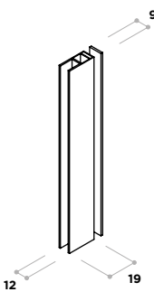
150000007 Cierre de imán angular adhesivo
