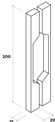
02010382 Tirador cube 20 Zamak
