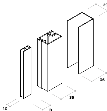
150000037 Cierre imán frontal a pared Access 150000038
