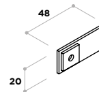
02010633 Aleta vierteaguas corredera Aluminio
