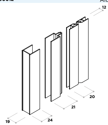
02020001 Cierre de imán angular 90° 02020019
