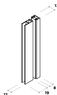
150000002 150000034 Cierre de imán frontal con perfil de aluminio a pared
