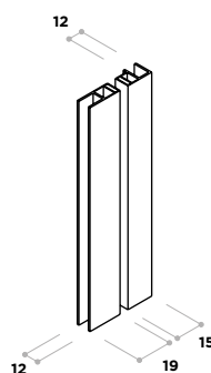
02020003 02020021 Cierre de imán angular lateral fijo
